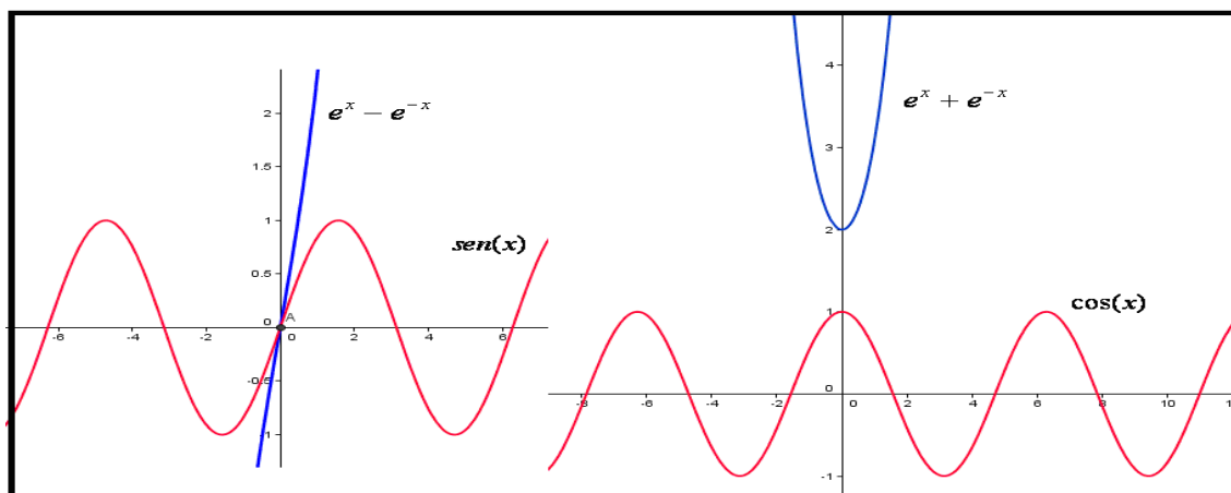
Figura 2: Identificação geométrica para a aplicação da regra de L'Hôpital
