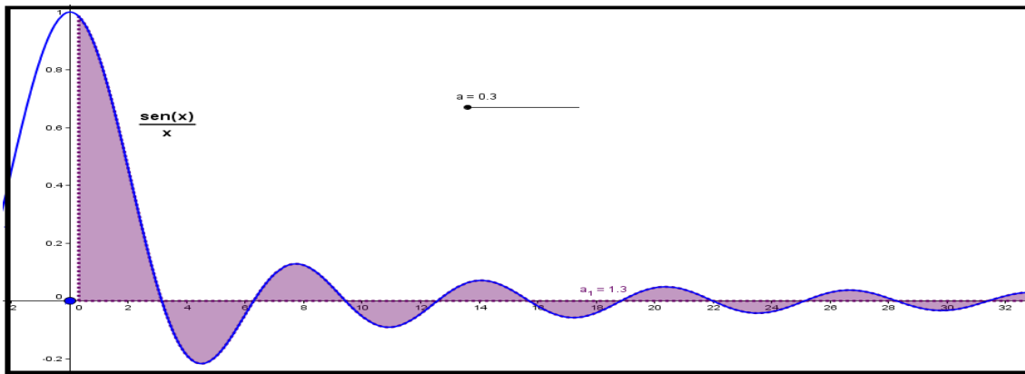
Figura 2: Interpretação geométrica do comportamento da integral imprópria e sua convergência O resultado que garante a produção de uma ilusão a respeito do comportamento da integral J_3 é evidenciado a partir do enunciado do seguinte teorema, demonstrado em Hairer & Wanner (2008, p. 259). Apresentamos, pois, seu enunciado.
