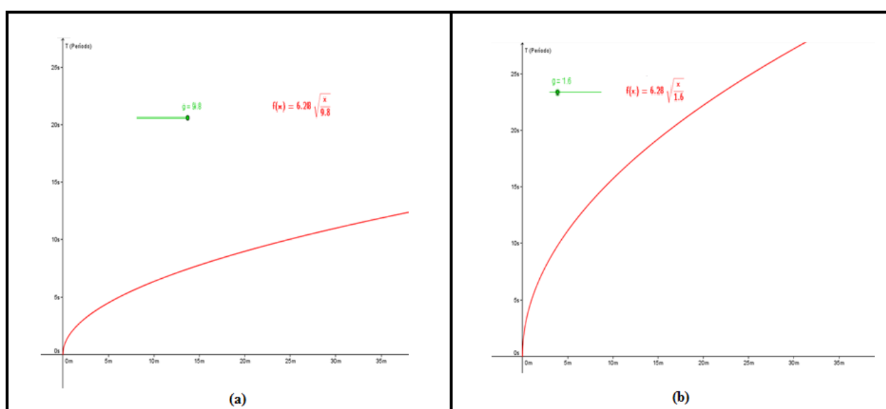
Figura 5: Comportamento gráfico da equação do período do pêndulo para (a) g = 9,8 \text{ m/s}^2 e (b) g = 1,6 \text{ m/s}^2 .
